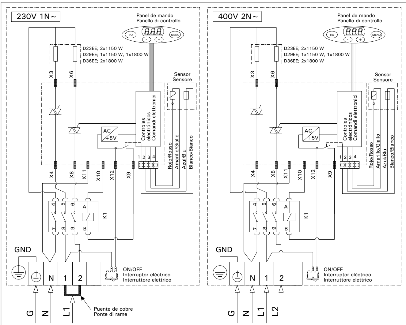
Figura 9a. Conexión de la fase 1 del calentador Figura 9a. Collegamento monofase della stufa
